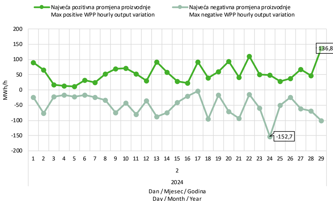
Slika 9 Maksimalna pozitivna i maksimalna negativna promjena satne proizvodnje VE u veljači 2024. godine
