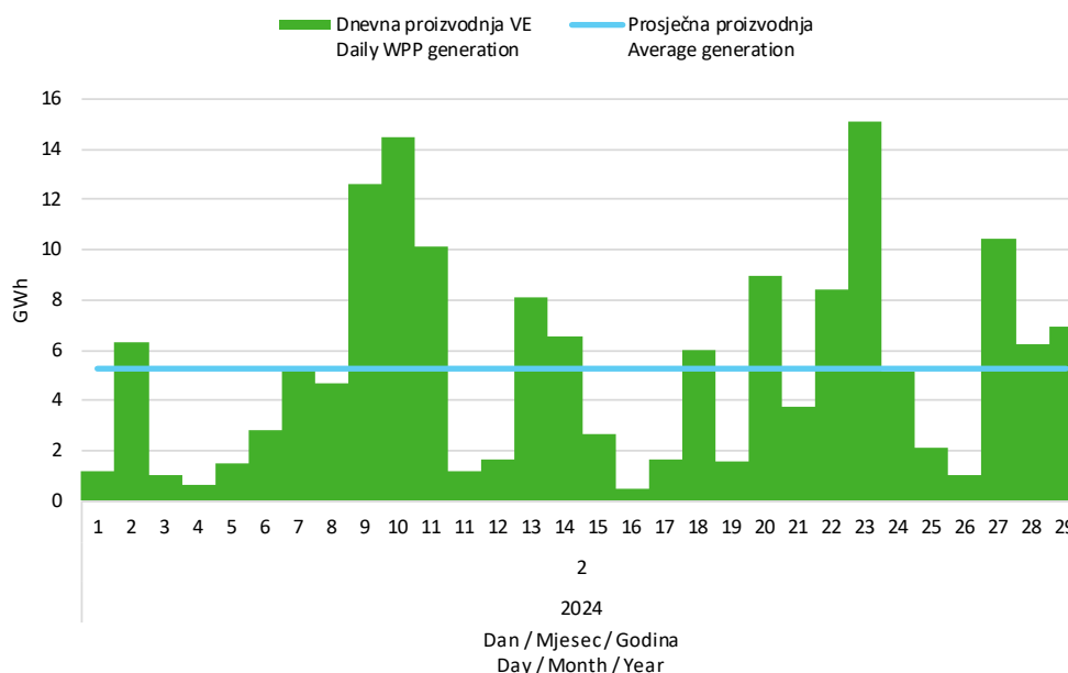
Slika 5 Dnevna proizvodnja svih vjetroelektrana u veljači 2024. godine
