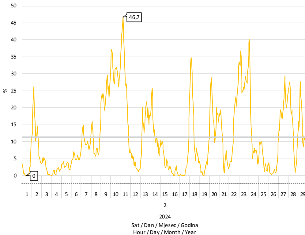
Slika 8 Udio proizvodnje vjetroelektrana u pokrivanju satnog opterećenja elektroenergetskog sustava u veljači 2024. godine
