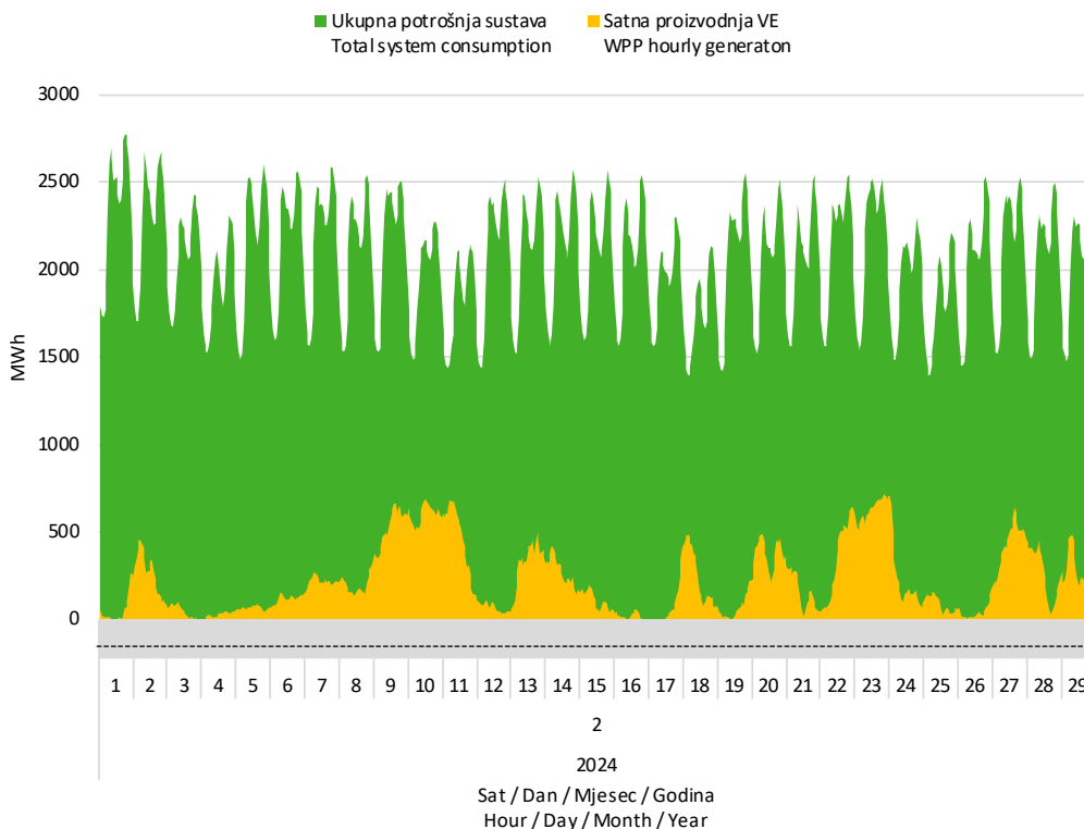
Slika 7 Usporedba satnog dijagrama opterećenja sustava i proizvodnje vjetroelektrana u veljači 2024. godine
