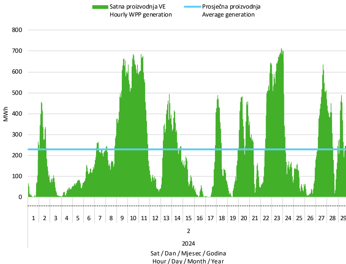
Slika 2 Satna proizvodnja svih vjetroelektrana u veljači 2024. godine Figure 2 Hourly generation of all wind power plants in February 2024
