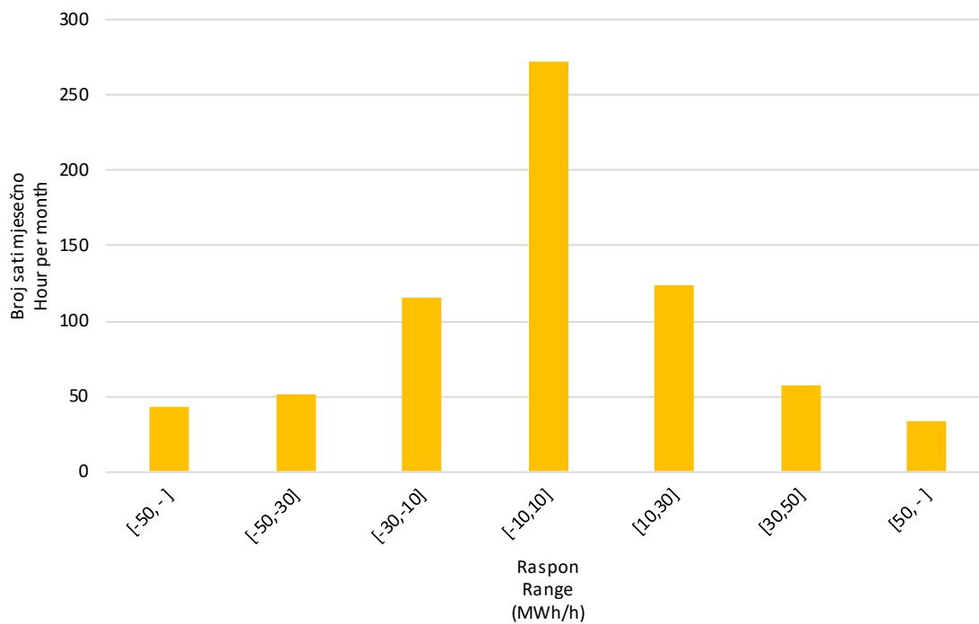
Slika 10 Statistička raspodjela satnih promjena proizvodnje VE u veljači 2024. godine
