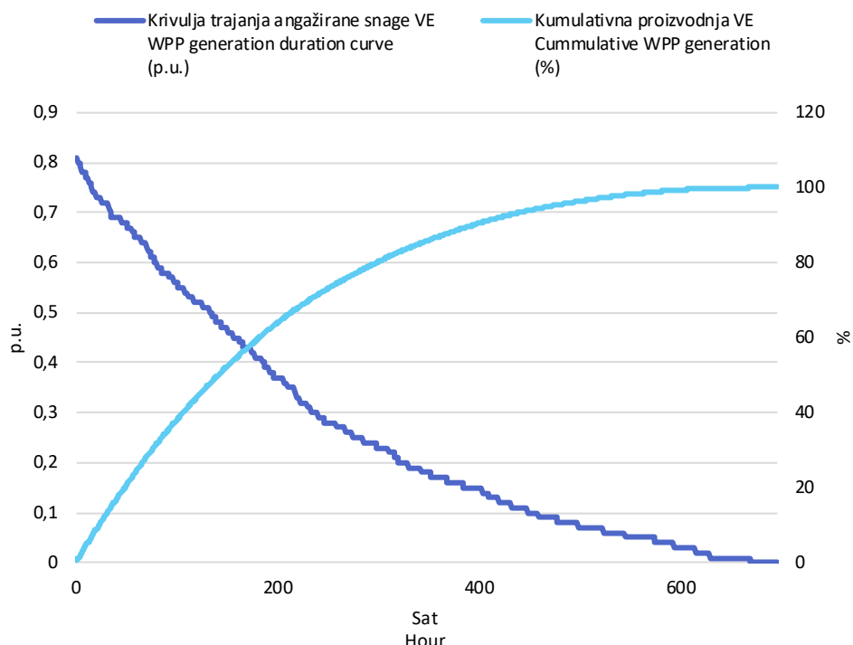
Slika 3 Krivulja trajanja angažirane snage svih VE i kumulativna proizvodnja VE u veljači 2024. godine u jediničnim vrijednostima
