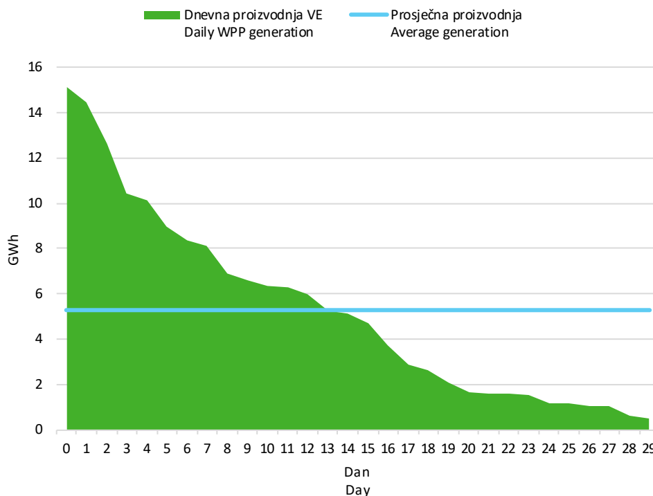
Slika 6 Krivulja trajanja dnevne proizvodnje vjetroelektrana u veljači 2024. godine
